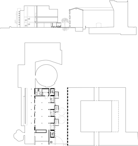
plantas i seccions peça · intervenció MACBA · plantas i seccions contextuais
